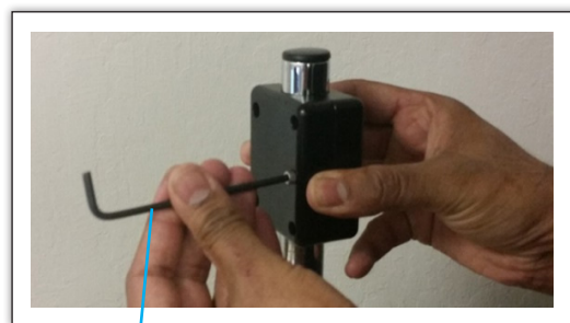
Chiave a brugola (5/32")
