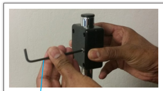
Unbrakonøkkel (5/32")
