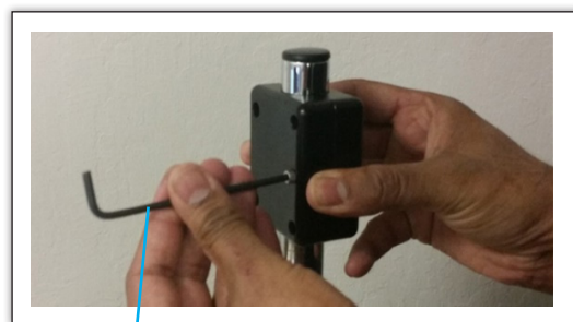
Unbrakonøgle (5/32 tomme)
